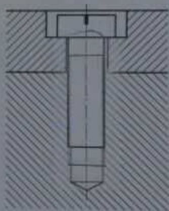
1-3补全螺钉连接图
